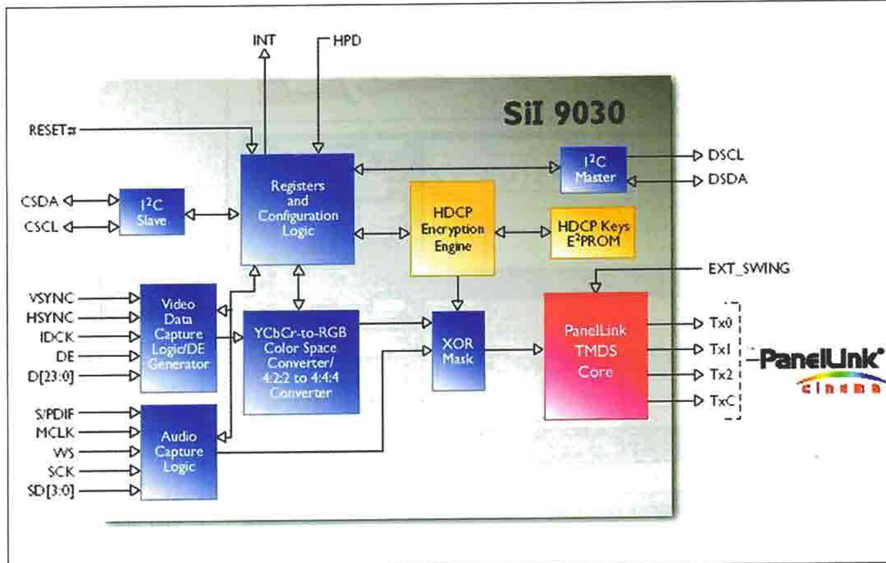
Schema a blocchi del trasmettitore HDMI Silicon Image Panellink SiI 9030.
