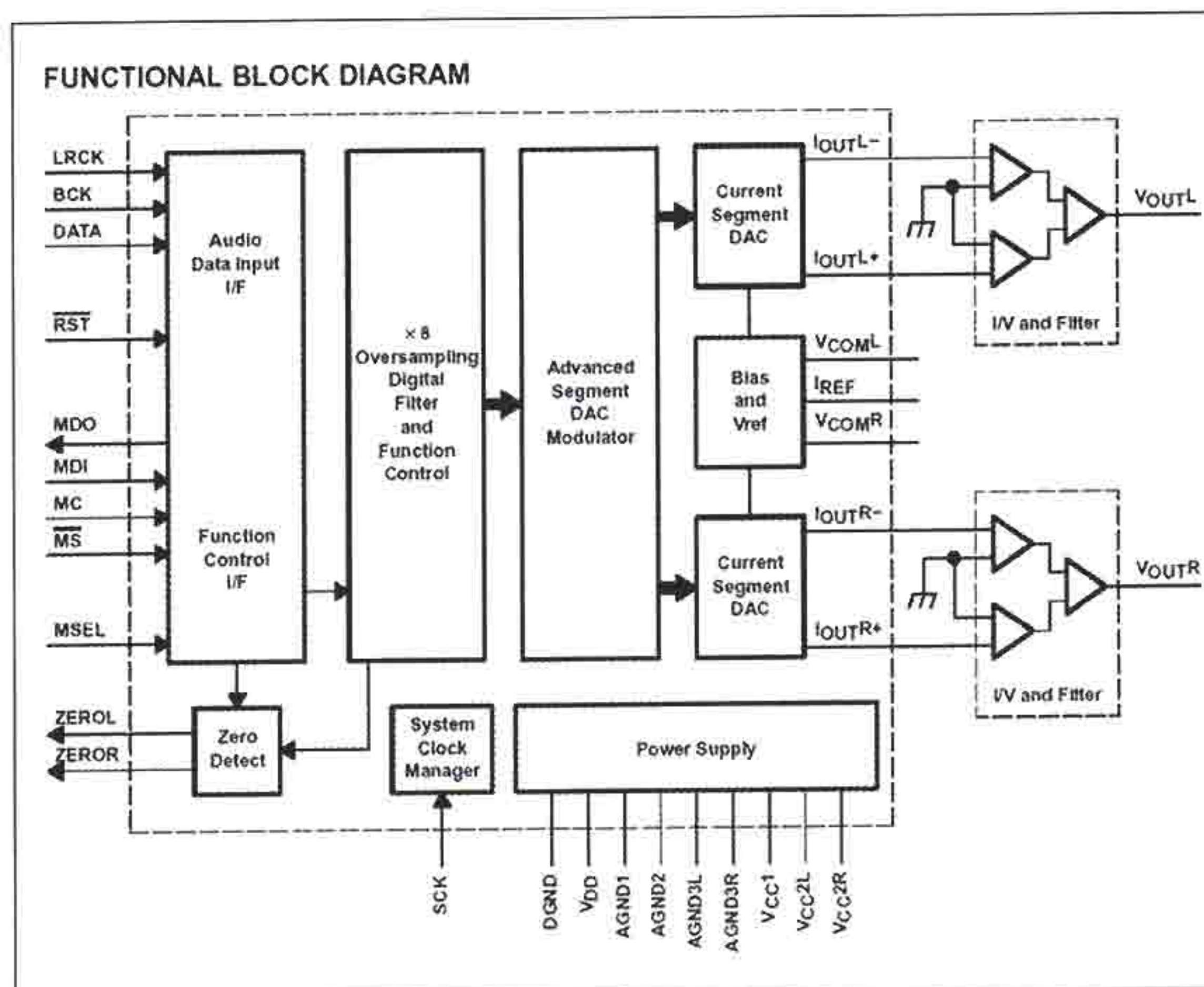
Schema a blocchi del convertitore D/A audio PCM 1796.
