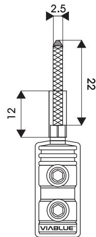
ViaBlue TS flexible pins item-no. 30212
