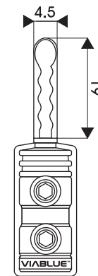
ViaBlue TS2 banana plug item-no. 30205
