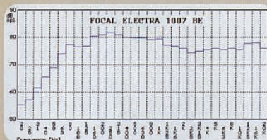
La linéarité du tweeter est exemplaire, le grave étant ici légèrement relevé pour cause d'évent débouchant en face arrière.
