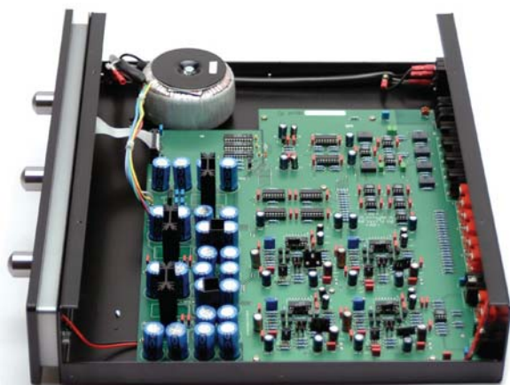
L'interno del pre è realizzato in modo ordinatissimo, quasi senza cablaggi; adottati sia componenti discreti sia numerosi circuiti integrati.
